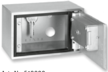
Art.-Nr. 510000 mit KRUSE-VdS-Umstellverschluss
