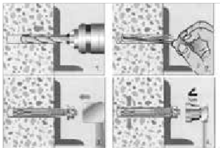
Abb. 3: Einbauanleitung Segmentanker
