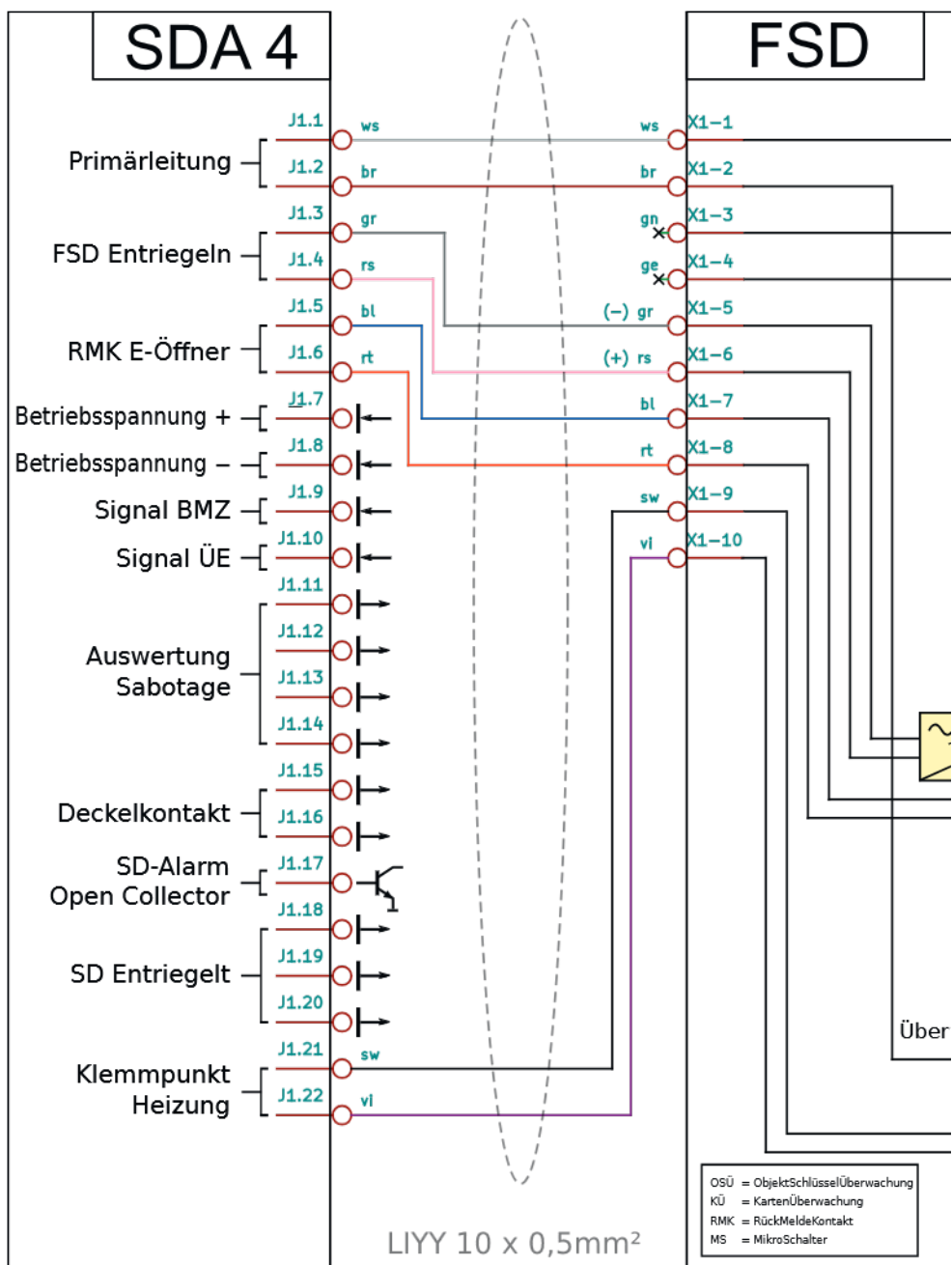
Anschlussplan
